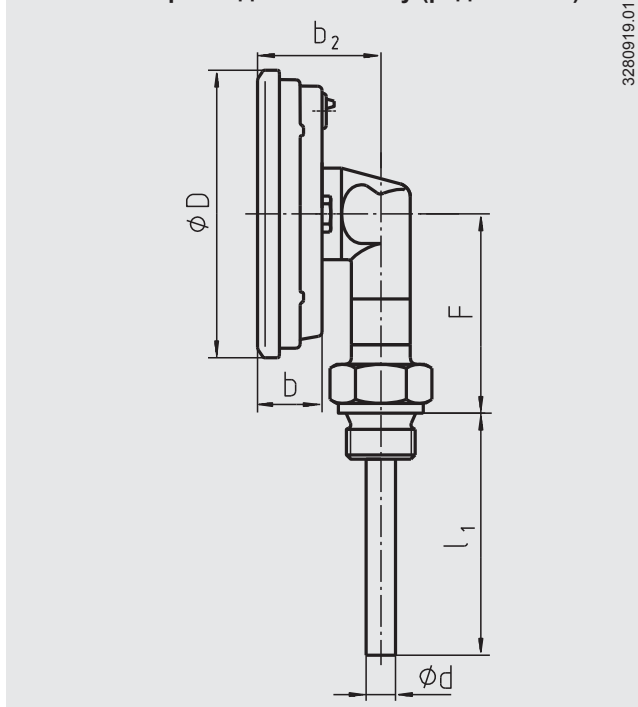
Положение присоединения снизу (радиальное)
