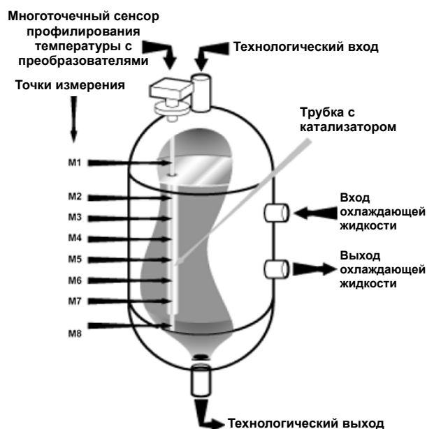
Рис. 1. Реактор
