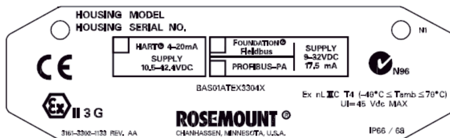
Табличка корпуса типа n
