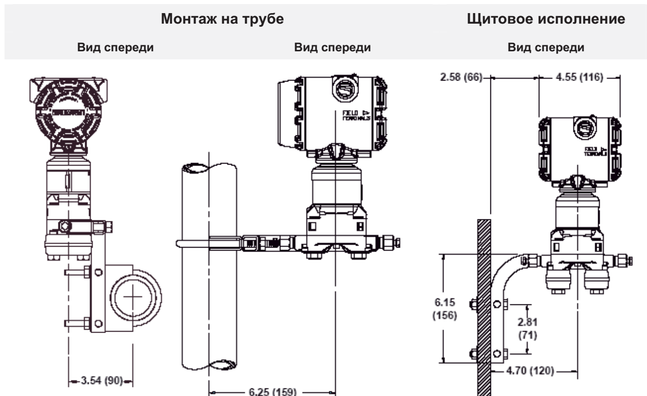
Рис. В-4. Монтажная компоновка Coplanar (кронштейн В4)
