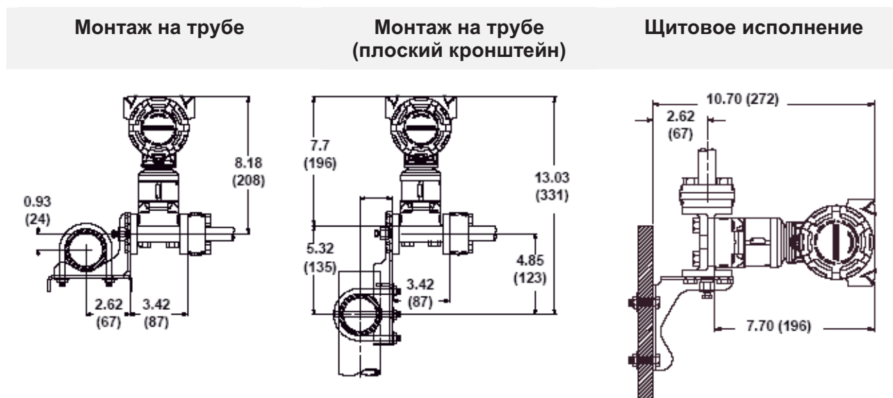
Рис. В-5. Стандартная монтажная компоновка
