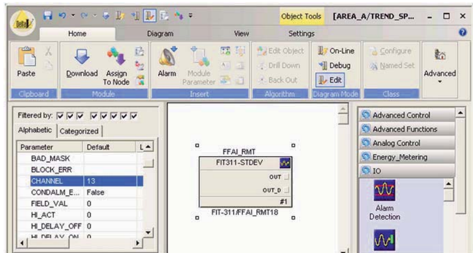
Рис. 6-12. Пример использования функционального блока AI для анализа стандартного отклонения в системе DeltaV
