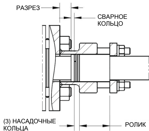
Рис. 2-25 иллюстрирует вид Annubar Flange-Lok по завершении установки. Пожалуйста, обратите внимание, что между корпусом Flange-Lok и сварным кольцом должен быть зазор.
