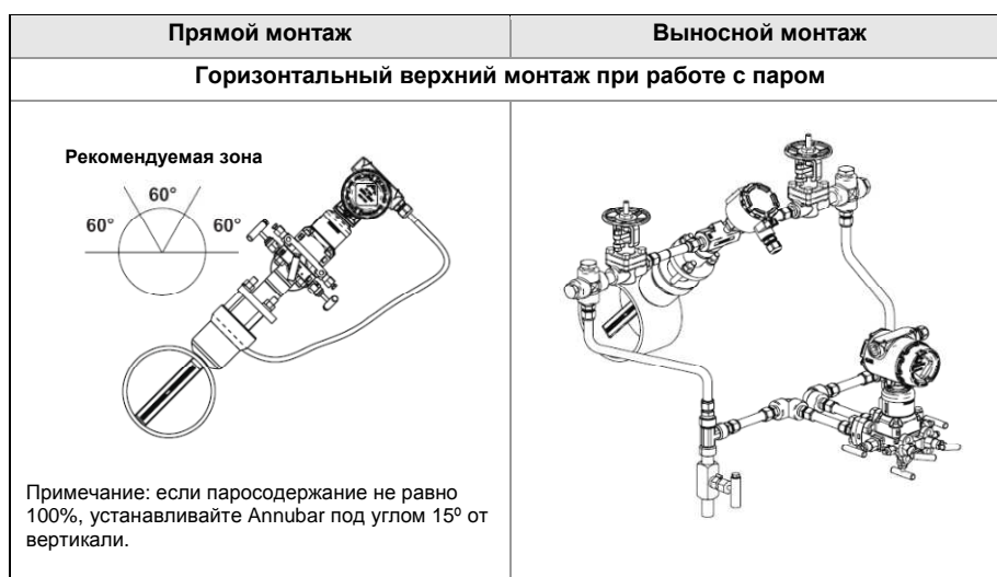
Рис. 2-8. Верхний монтаж при работе с паром
