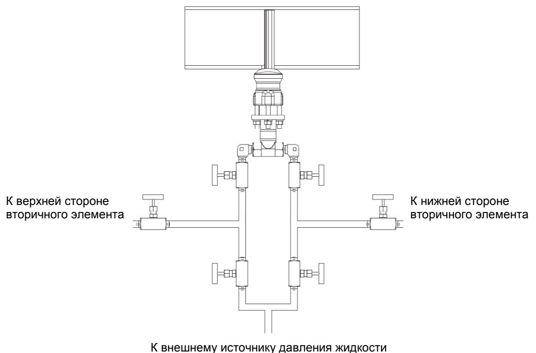
Рис. 4-4. Схема импульсного трубопровода для продувки
