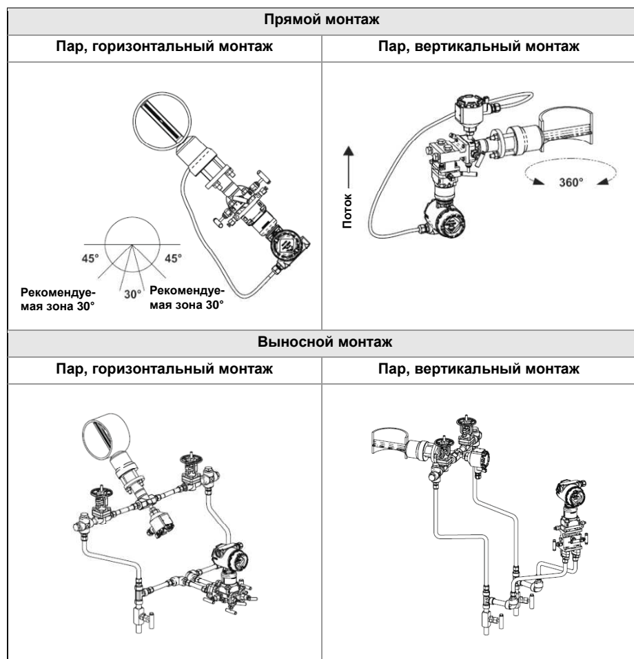
Рис. 2-7. Применение с паром
