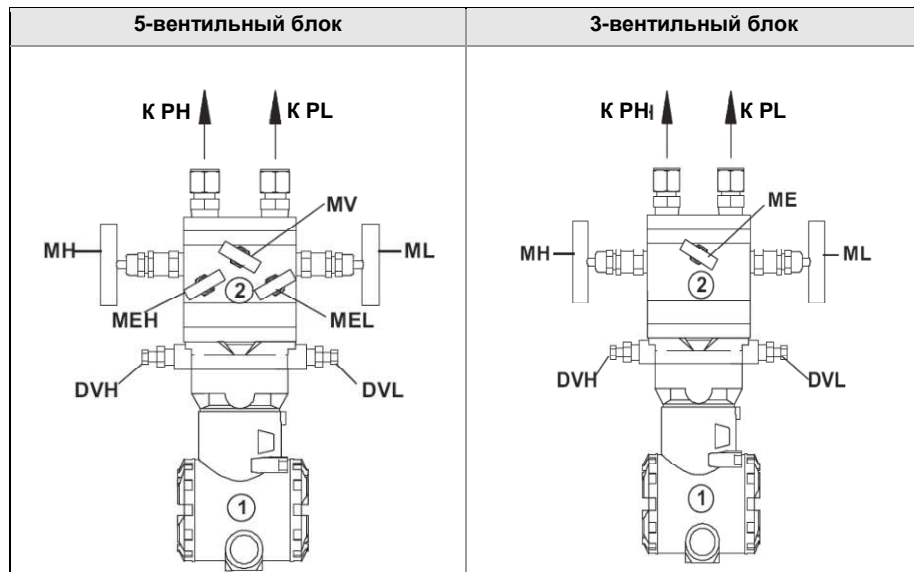
Рис. 2-3. Идентификация вентилей для 5- и 3- вентильных блоков
