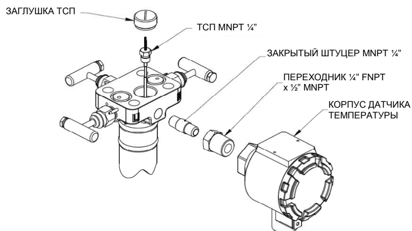
Рис. 4-1. Annubar с прямым монтажом и встроенным ТСП в разобранном виде
