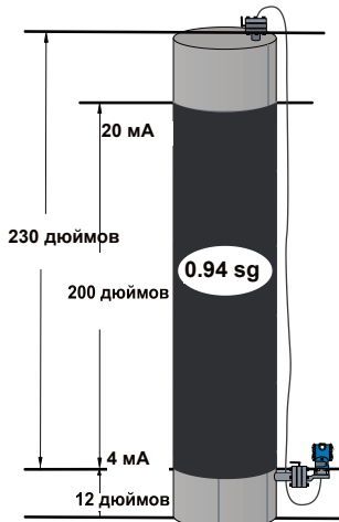
Рис. 3-9. Пример резервуара
