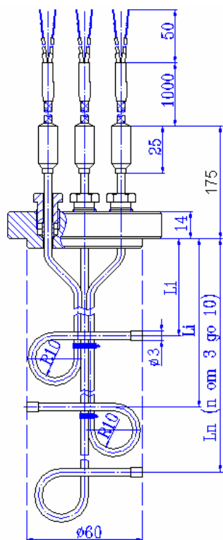
Рисунок Б.1 – ТХА Метран-261-01, ТХК Метран-262-01
